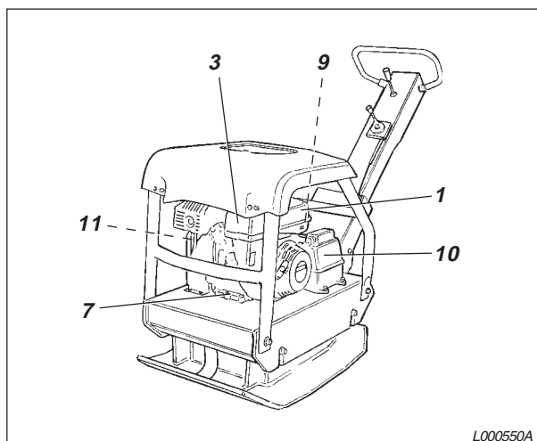
Fig. 2 MV 220/230/245
